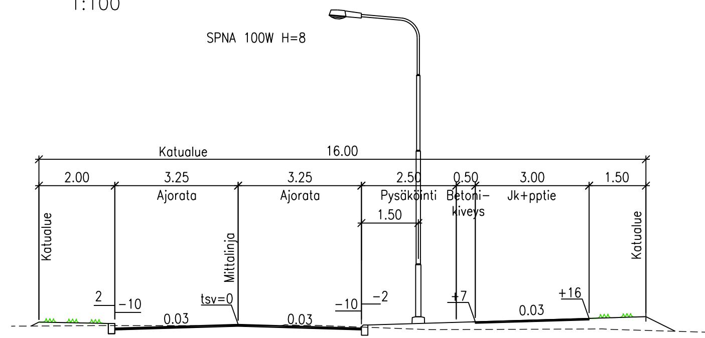
PAJATIE (PL 55) TYYPIPOIKKILEIKKAUS, AJORATA+JKPPTIE 1:100
