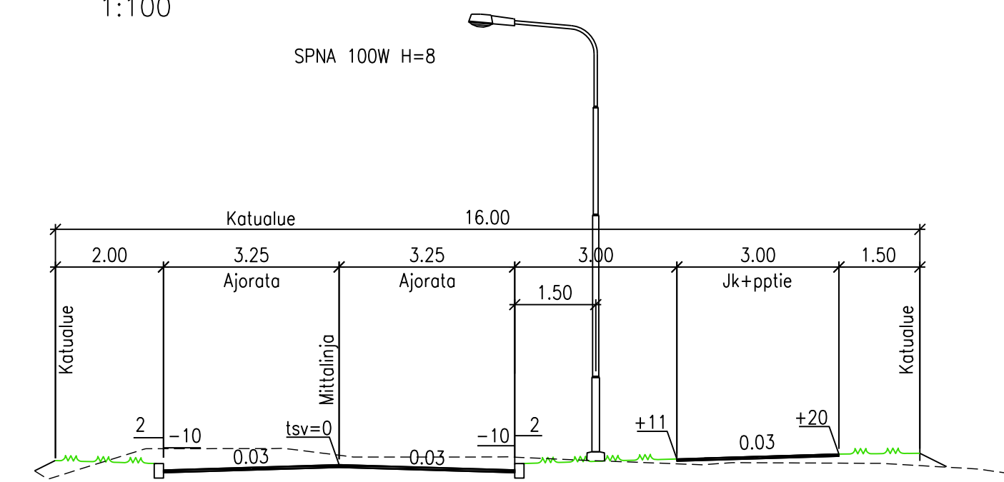
PAJATIE (PL 220) TYYPIPOIKKILEIKKAUS, AJORATA+JKPPTIE 1:100
